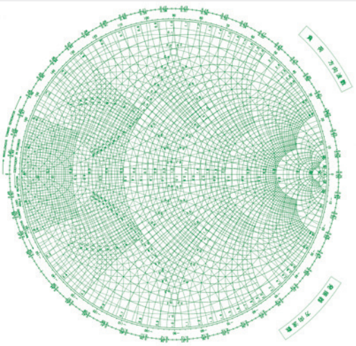
A4-I2 イミッタンスチャート
