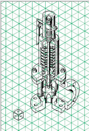
アイソメトリック図法による投影図
