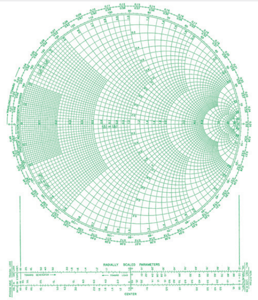
A4-ス52 スミスチャート（インピーダンスチャート）
